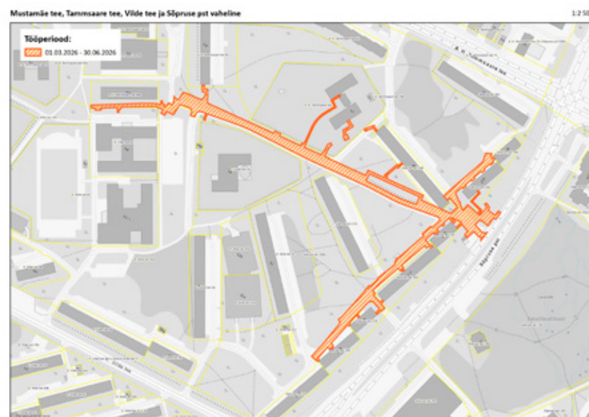
Skeemid „Rekonstrueeritav soojustorustik Ehitajate tee, Sütiste tee ja Sõpruse pst ning Mustamäe tee, Tammsaare tee, Vilde tee ja Sõpruse pst vahelises piirkonnas“.
